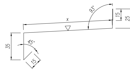
O05 Vodorovné dolní zpracování okna
