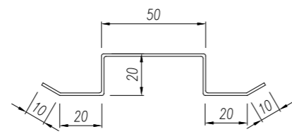
P01 Profil střední 20/50
