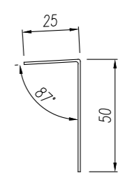
O06 Podpěra vodorovného dolního zpracování okna
