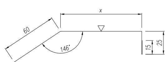
O04 Vodorovné horní zpracování okna
